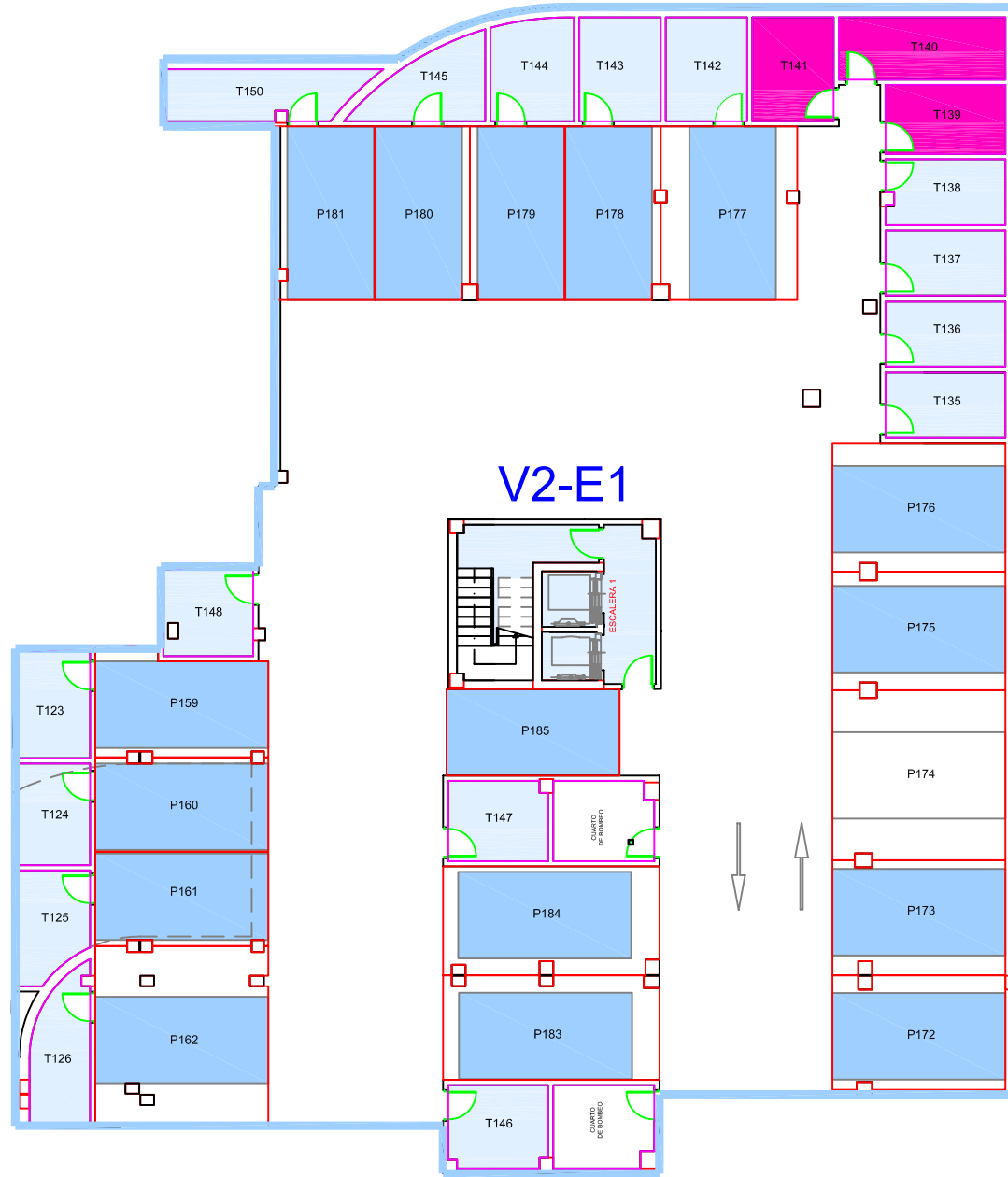
SÓTANO NIVEL 2 V2 - E1 COOPERATIVA PARQUE PRÍNCIPE FASE I
